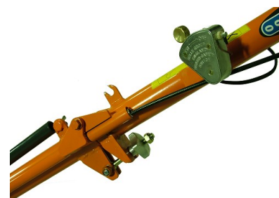
Inklapbare handgreep
